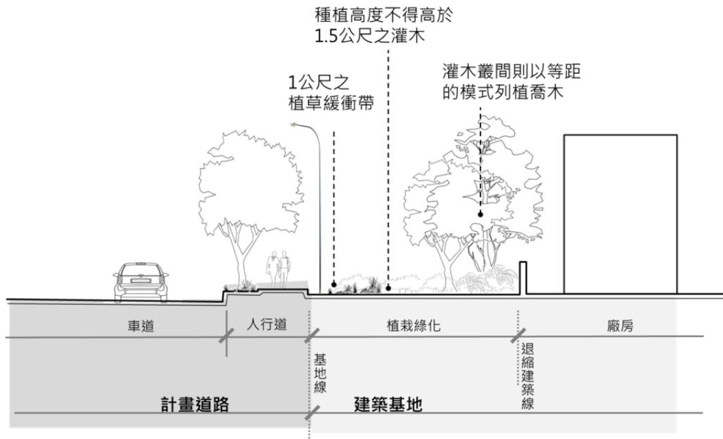
臨計畫道路之建築基地退縮示意
