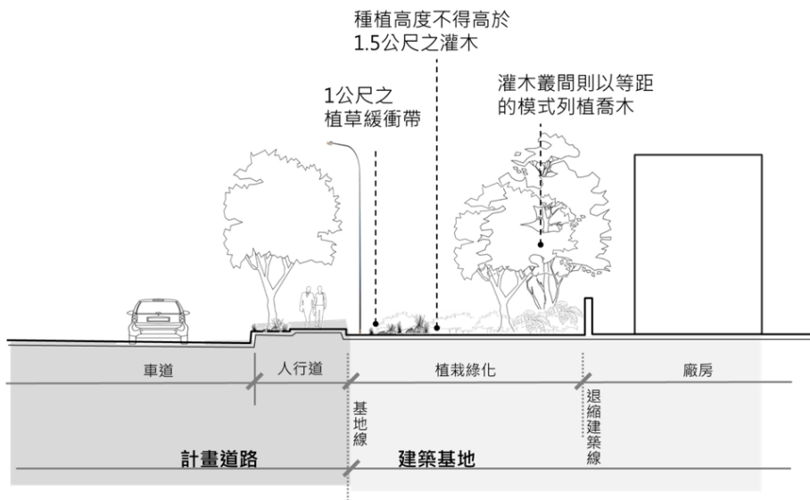
圖 5-6 臨計畫道路之建築基地退縮示意圖
